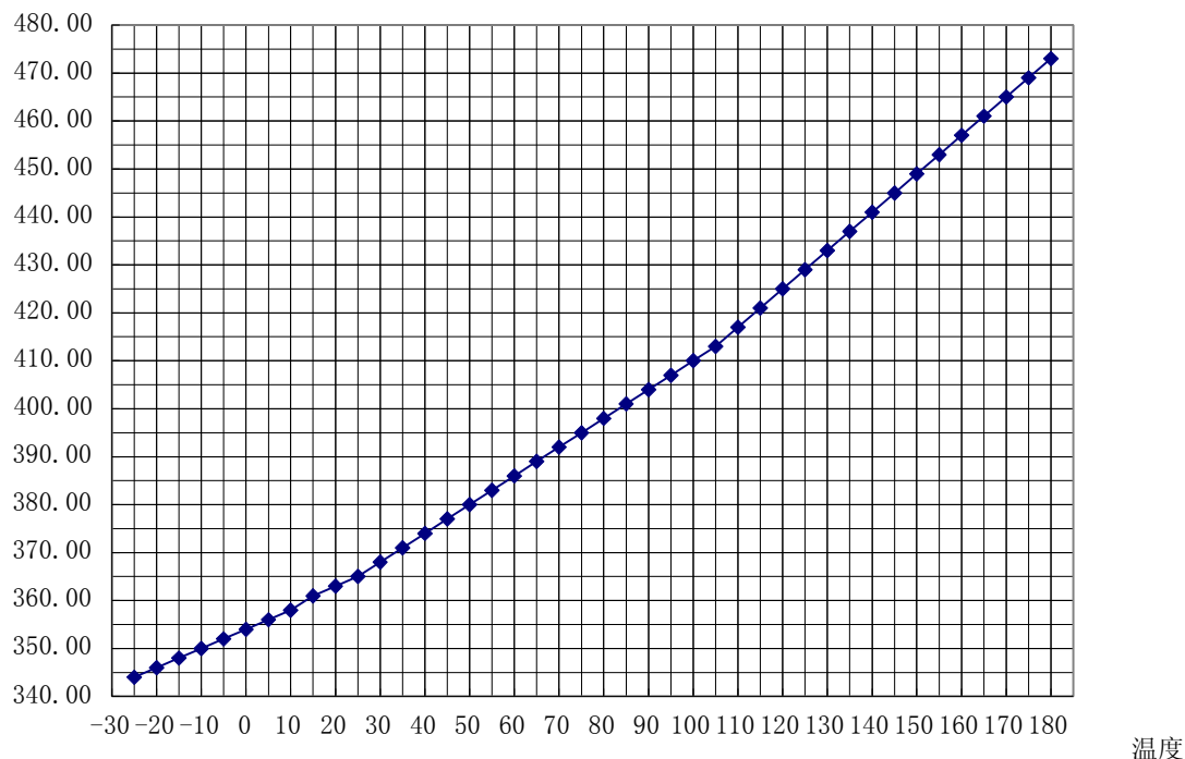
温度—阻值曲线图
