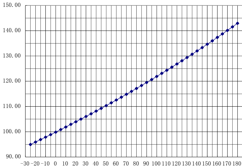
温度—阻值曲线图
