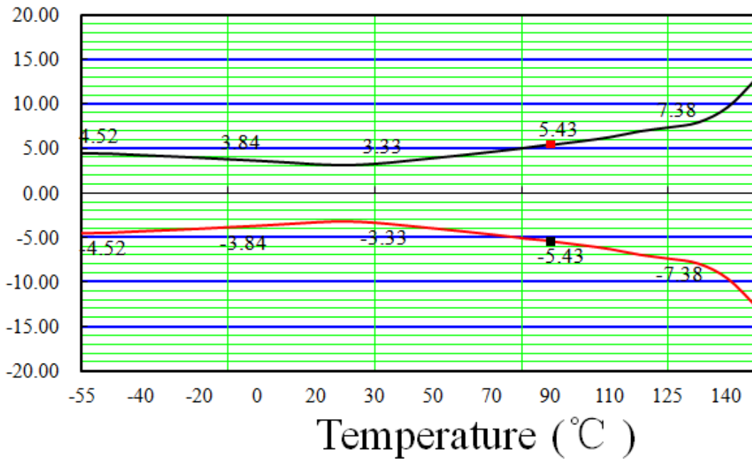
华巨电子KTY82-152测温最大偏差 °C
