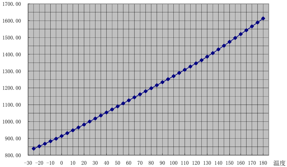
温度—阻值曲线图
